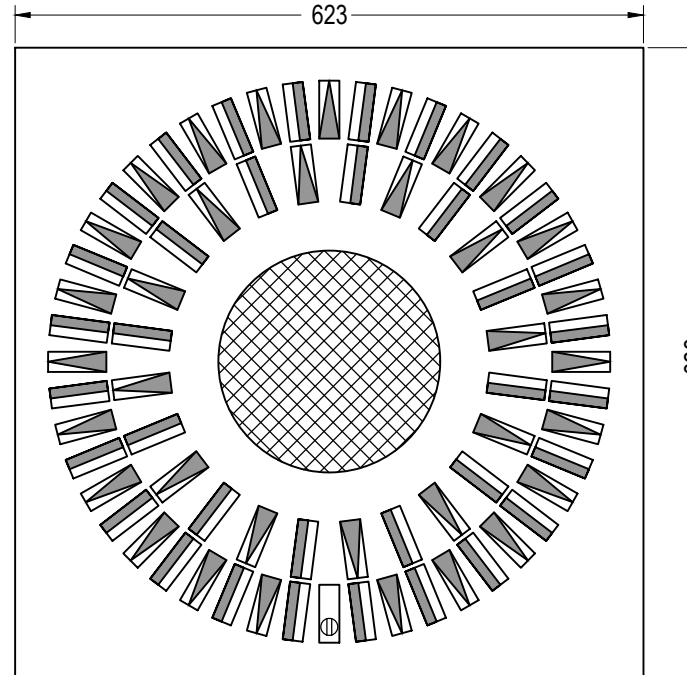
bottom view, scale 1:7,5
