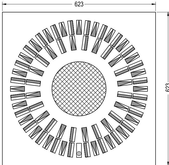
bottom view, scale 1:7,5
