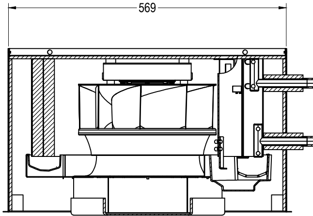
section B-B, scale 1:7,5
