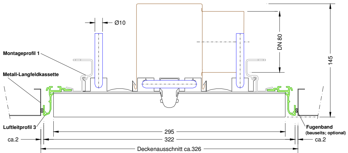
Schnitt A
