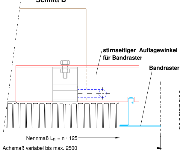
Schnitt B
