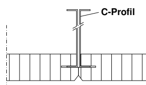
Schnitt C
