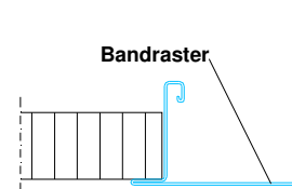
Schnitt D
