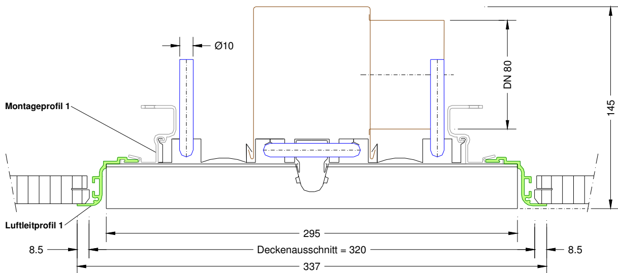
Schnitt A
