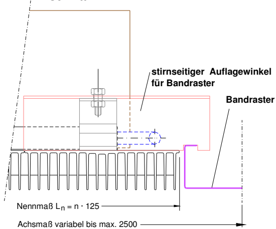
Schnitt B
